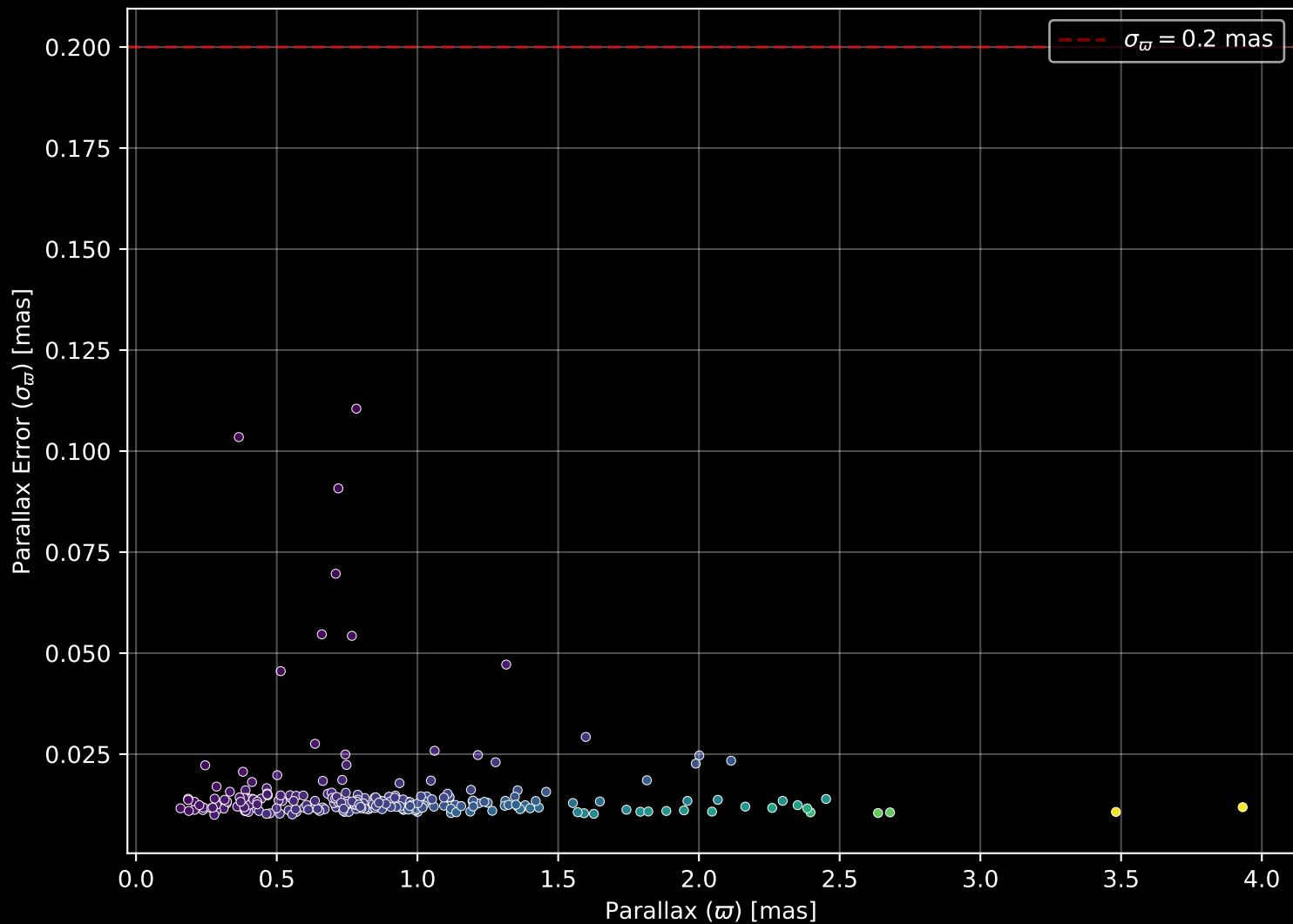
GALAH DR4 Field: [8390] Parallax Quality (n= 246)
