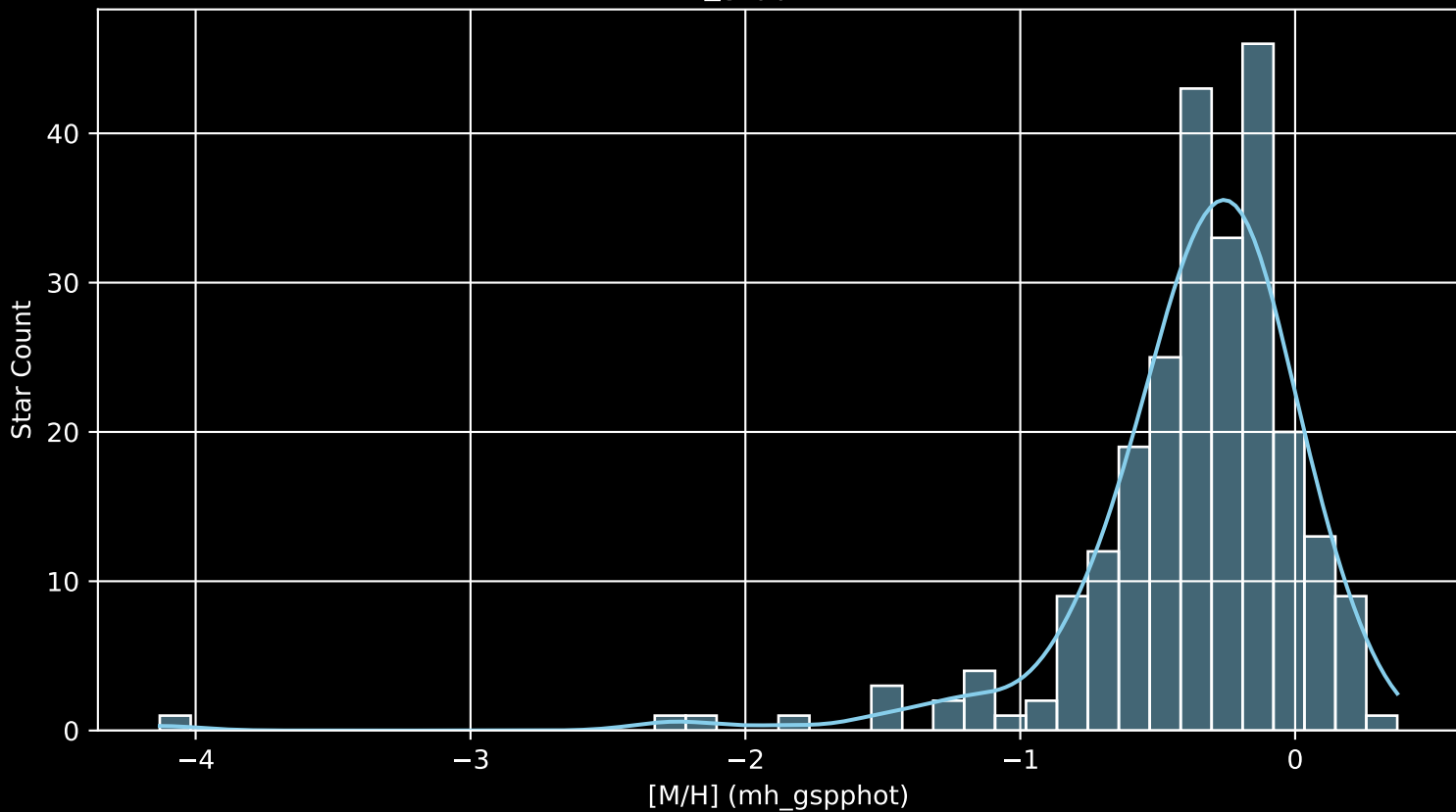
GALAH DR4 Field: [8390] [M/H] (mh_gspphot) (n= 246)
