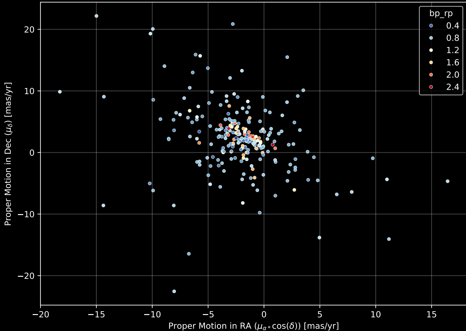
GALAH DR4 Field: [8390] Proper Motion Diagram (n= 246)
