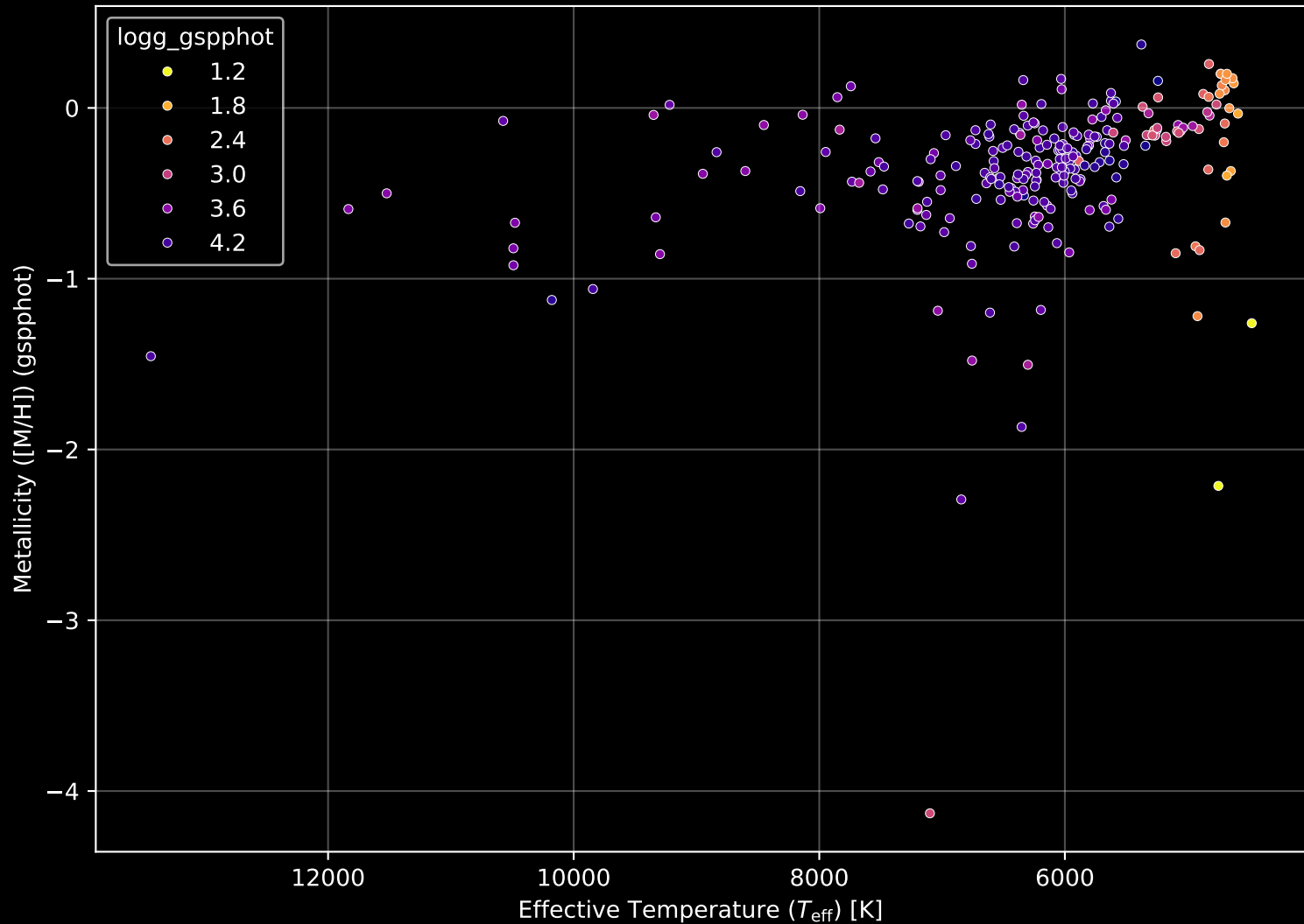
GALAH DR4 Field: [8390] Stellar Population Parameters (n= 246)
