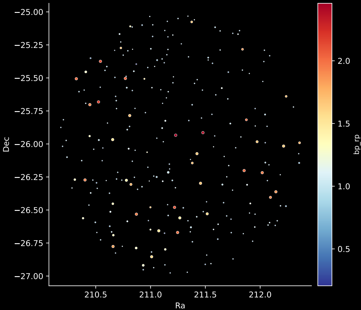
GALAH DR4 Field: [8390] Stars: 246
